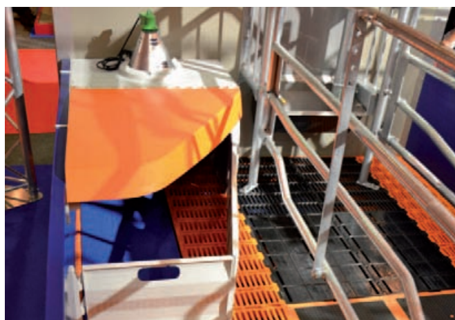
Figure 2 : Détail de l'aménagement au niveau d'une niche en maternité
