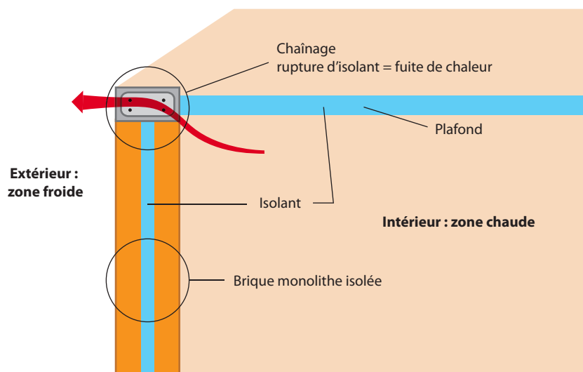
Exemple de ponts thermiques sur la zone de chaînage
