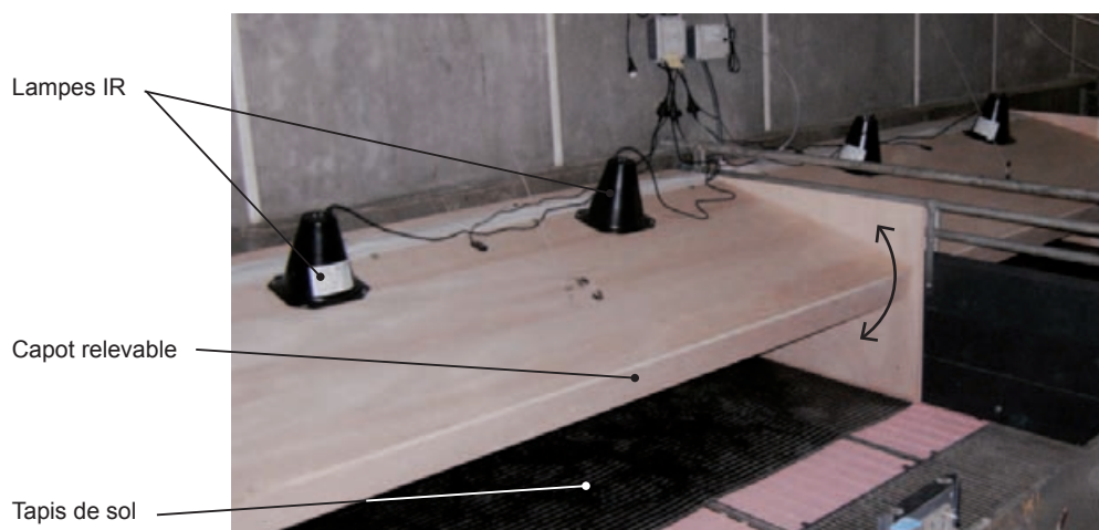
Figure 1 : Détail de l'aménagement au niveau d'une niche en PS
