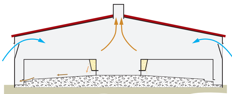
La ventilation naturelle
