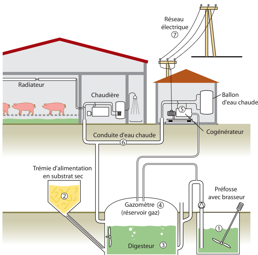
Synoptique de fonctionnement d'une installation de méthanisation agricole (dispositif en phase liquide infiniment mélangée)
