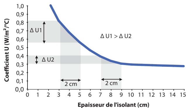
Évolution de U en fonction de l'épaisseur de l'isolant dans une paroi sandwich (polystyrène extrudé)
