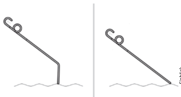
Figure 2 : Deux formes différentes de dents de herse étrille
