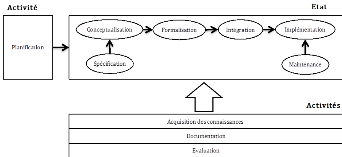
Figure 2 : Processus de développement d'ontologie avec METHONTOLOGY (source : Fernández-López, Gómez-Pérez et al., 1997)
